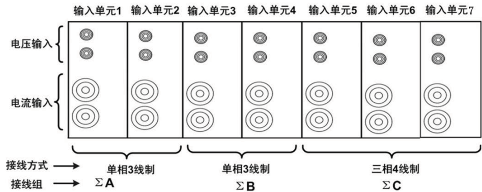
图 2.22 接线组
