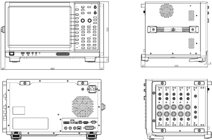
图 7.1 尺寸图
