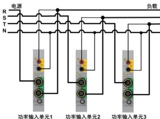
图 4.59 三相 4 线制接线实例
