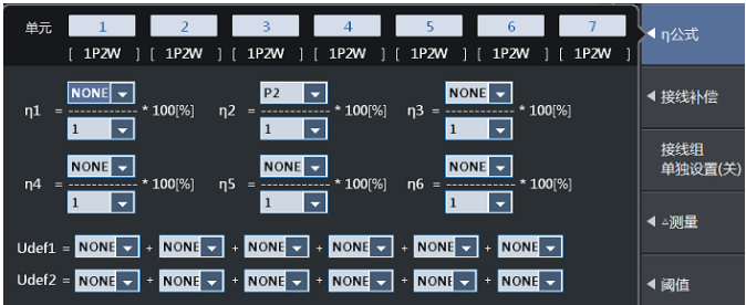
图 4.28 \eta 公式配置对话框
