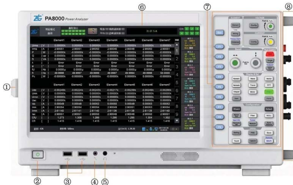
图 3.1 前面板
