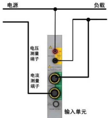
图 4.47 1P2W 下功率分析仪接线实例
