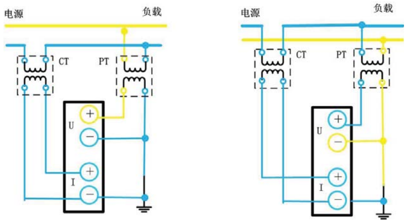
图 4.46 单相 2 线制(1P2W)，使用 PT/CT 时的接线举例
