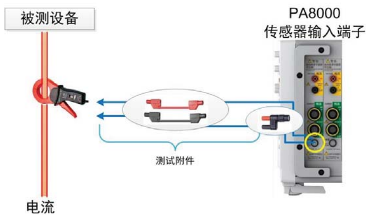
图 4.64 使用电压输出型传感器输入端子测量电流
