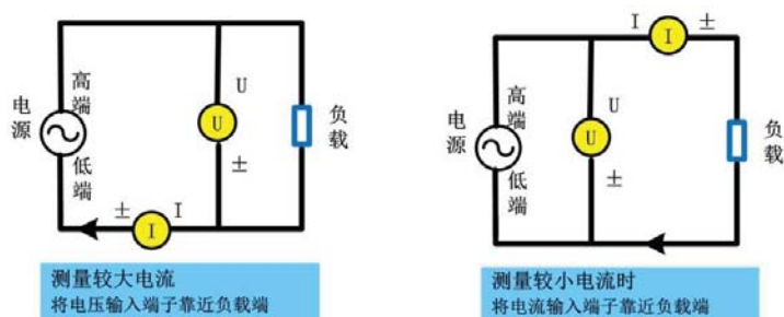
图 4.44 测量电压和电流的大小对测量的影响
