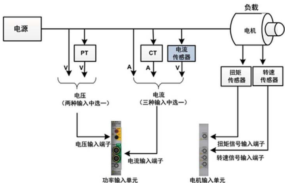
图 2.21 输入信号到输入单元
