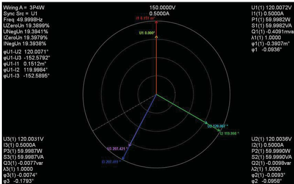
图 2.14 向量显示
