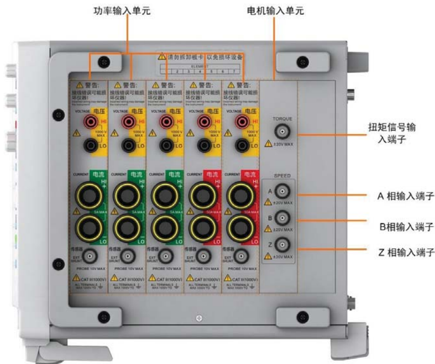
图 2.20 电机信号输入
