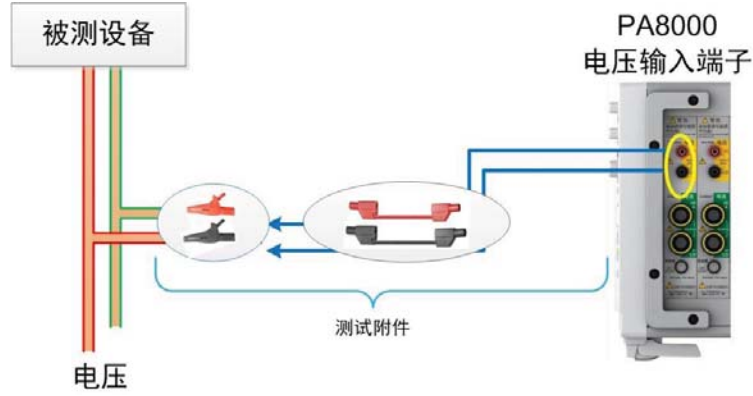
图 4.60 使用电压输入端子直接测量电压
