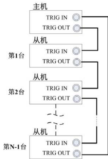
图 4.35 多台仪器级联示意图
