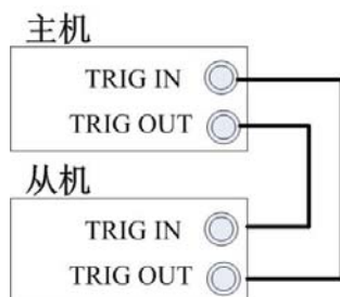
图 4.34 两台机器级联示意图
