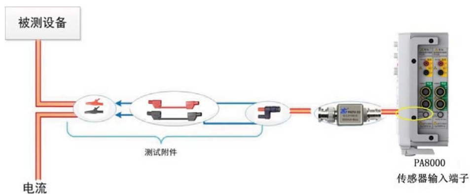
图 4.63 使用分流型传感器输入端子测量电流
