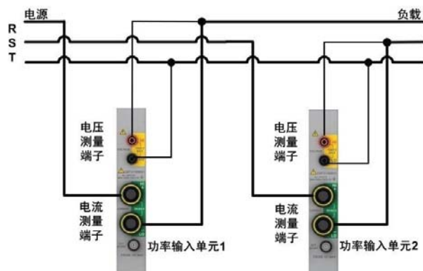
图 4.53 3P3W 下功率分析仪接线示例
