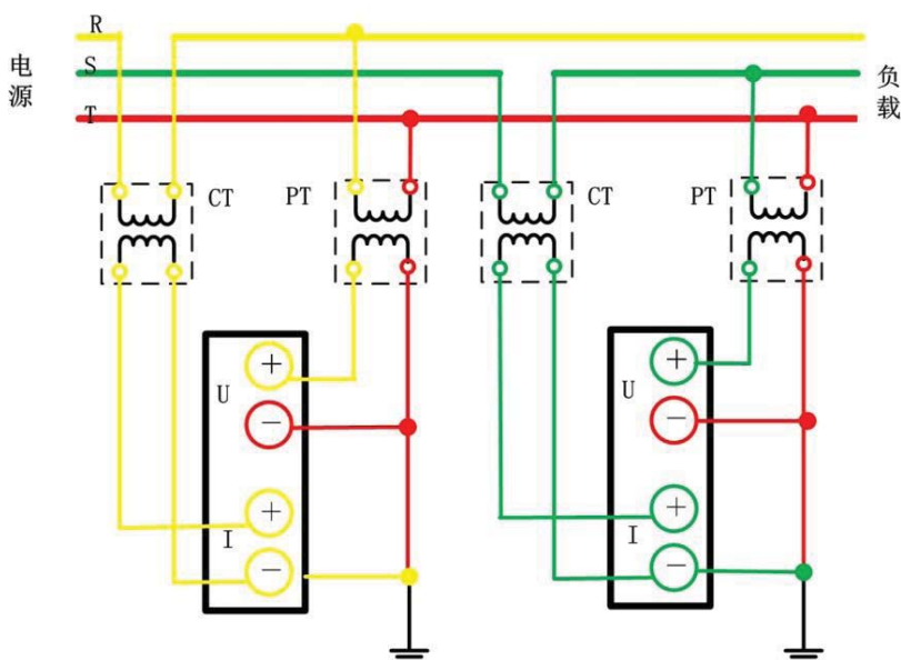
图 4.52 三相 3 线制(3P3W)、使用 PT/CT 时的接线举例
