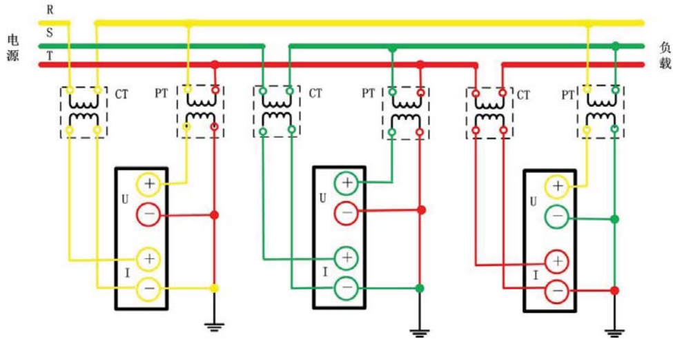
图 4.55 三相 3 线制 (3 电压 3 电流表法), 使用 PT/CT 的接线
