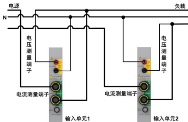
图 4.50 1P3W 下功率分析仪接线实例
