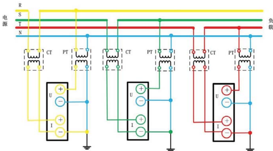
图 4.58 三相 4 线制(3P4W)、使用 PT/CT 时的接线举例
