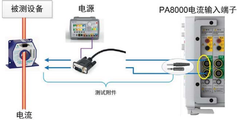
图 4.62 使用电流传感器（CT）和电流输入端子测量电流
