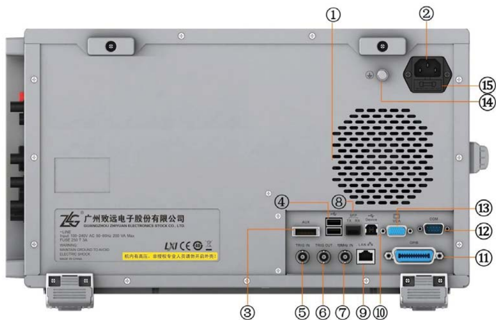
图 3.25 后面板说明
