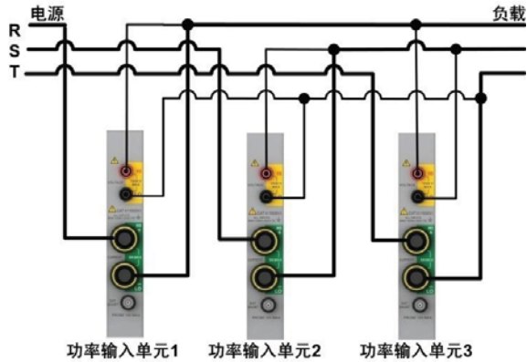
图 4.56 3P3W (3 电压 3 电流表法) 下功率分析仪接线示例
