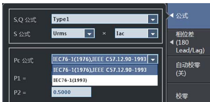
图 4.26 选择 Pc 公式
