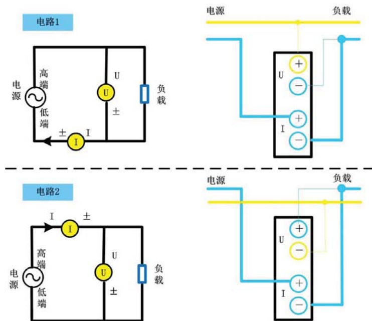
图 4.45 单相 2 线制(1P2W)，测量仪表的接线
