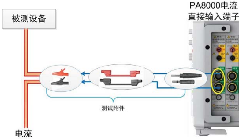
图 4.61 使用电流输入端子直接测量电流
