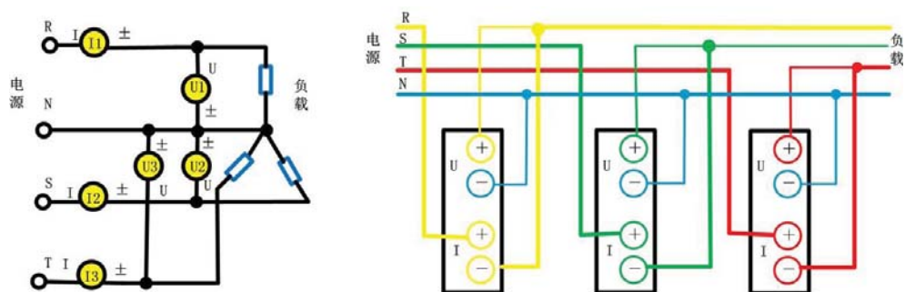
图 4.57 三相 4 线制下的测量仪表接线
