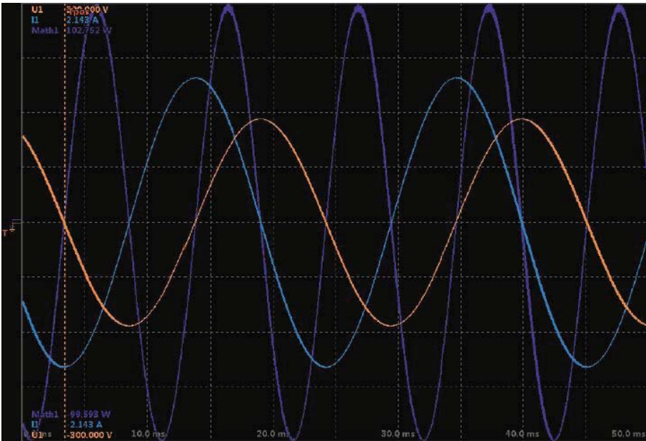
图 2.18 波形运算
