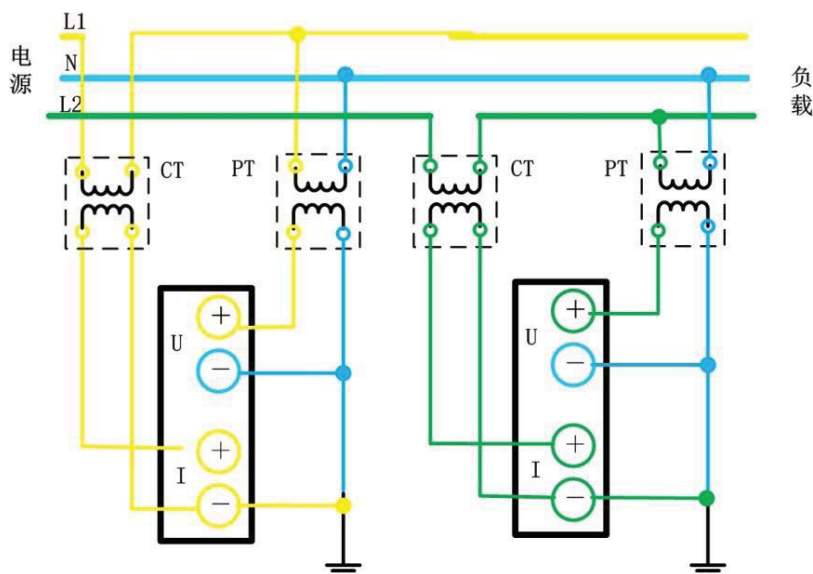
图 4.49 单相 3 线制(1P3W)、使用 PT/CT 时的接线示例
