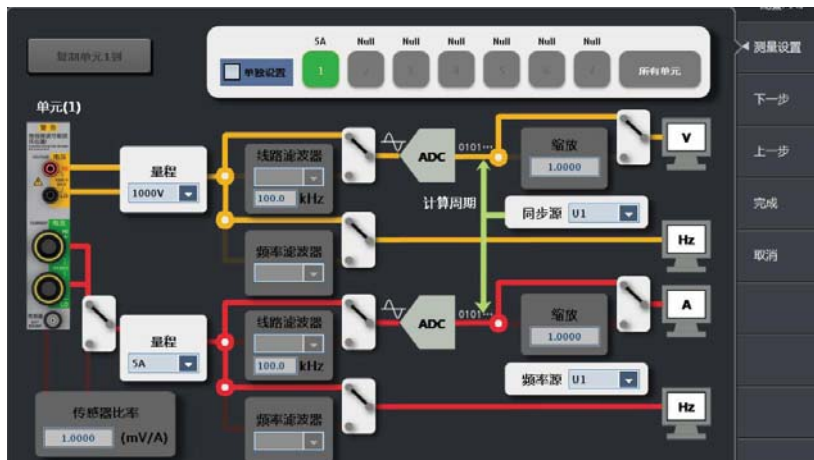
图 3.3 配置向导之测量图片
