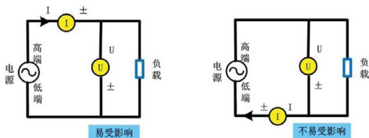
图 4.43 降低杂散电容对测量精度的影响
