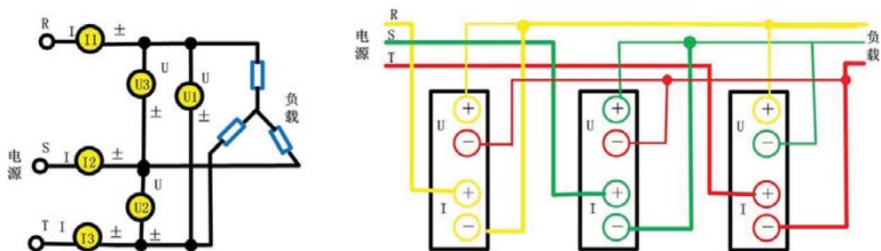
图 4.54 三相 3 线制（3 电压 3 电流表法），测量仪表接线
