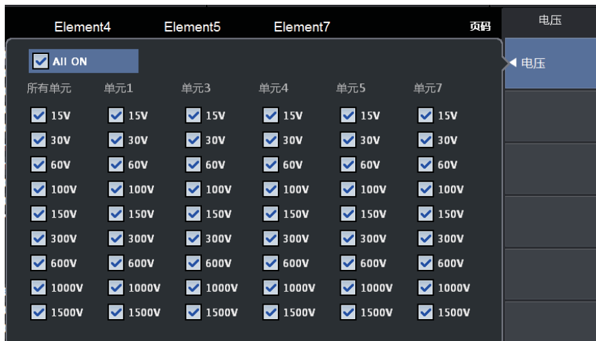
图 3.11 PA8000/PA6000H 电压量程范围配置
