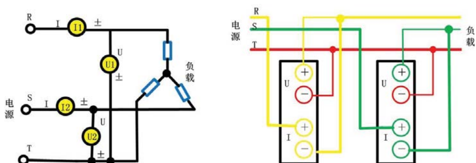
图 4.51 三相 3 线制、测量仪表的接线
