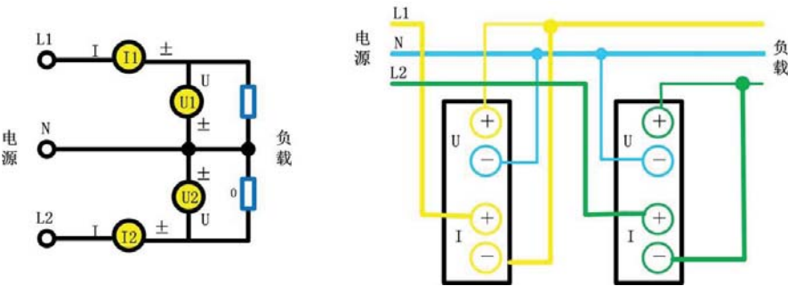
图 4.48 单相 3 线制(1P3W)，测量仪表的接线
