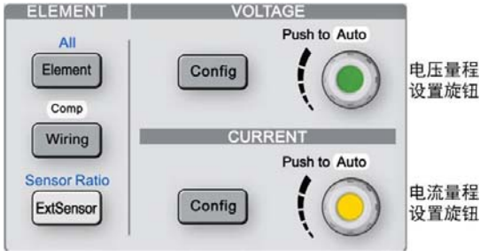
图 3.13 量程设置旋钮
